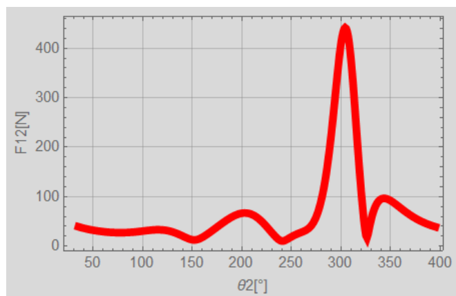
Figura 19: Gráfica de la fuerza 12
