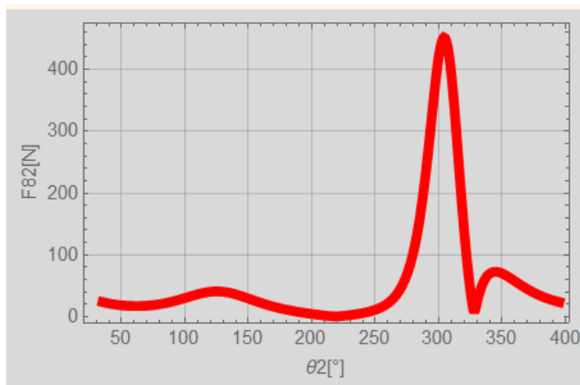
Figura 21: Gráfica de la fuerza 82
