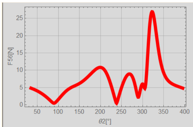
Figura 25: Gráfica de la fuerza 56
