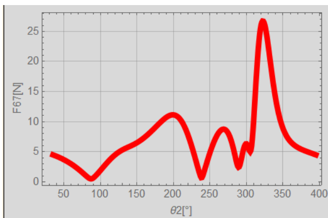
Figura 26: Gráfica de la fuerza 67
