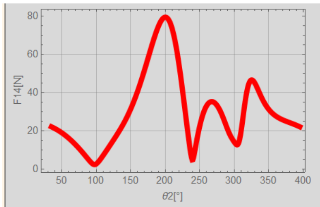
Figura 23: Gráfica de la fuerza 14
