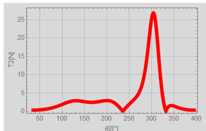
Figura 29: Gráfica del par de entrada en el cuerpo 2
