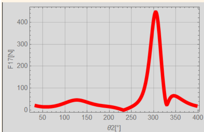
Figura 27: Gráfica de la fuerza 17
