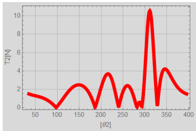
Figura 30: Gráfica del par de entrada en el cuerpo 2
