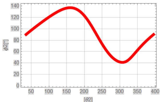
Figura 32: Ángulo de transmisión de los eslabones 4 y 5
