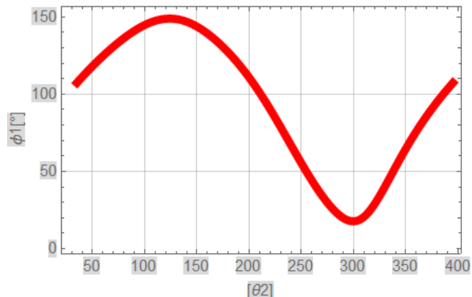
Figura 31: Ángulo de transmisión de los eslabones 6 y 7
