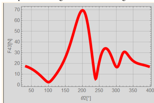
Figura 22: Gráfica de la fuerza 43
